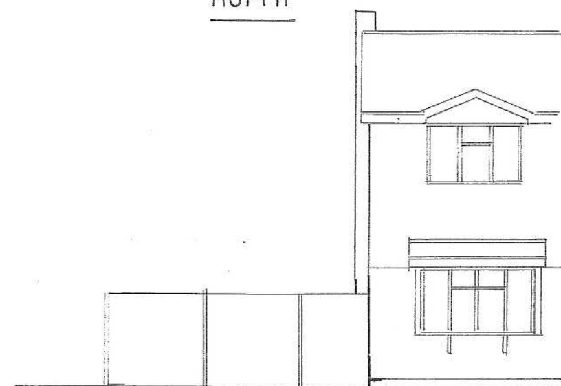
west 1 : 100
