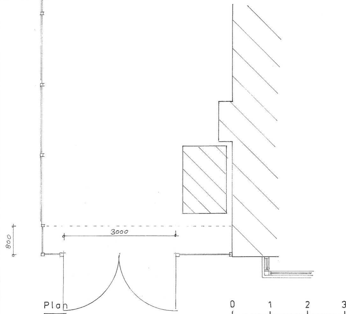
Plan 1 : 50 Existing
