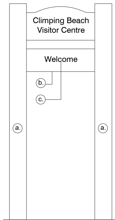
9. WELCOME SIGNAGE 1:20
