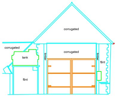
Elevation 1
