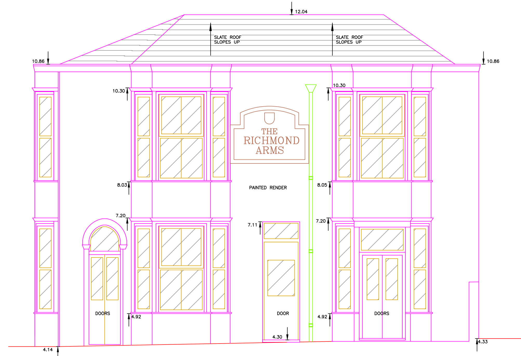
Elevation 2
