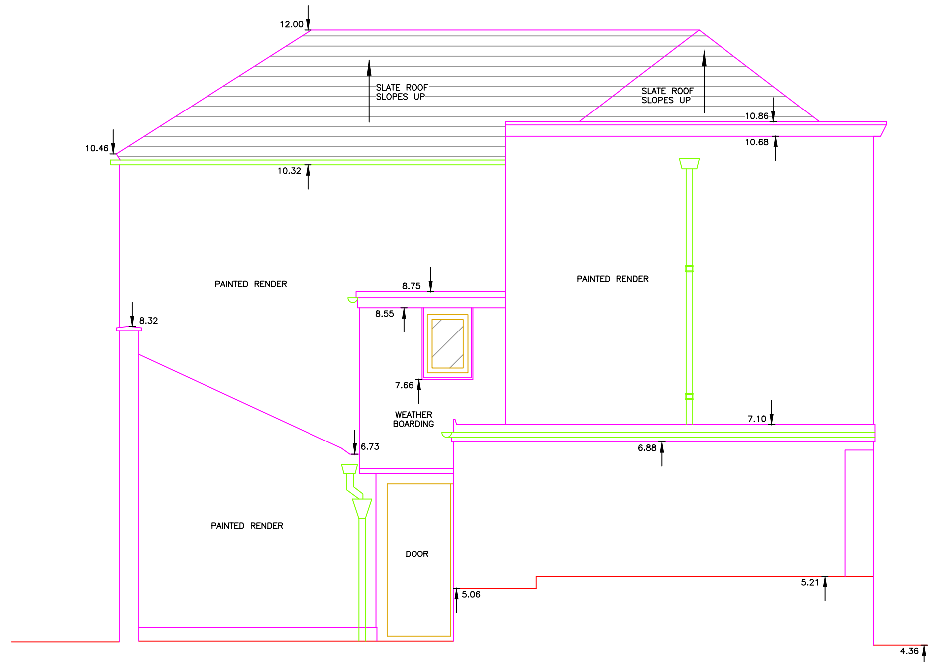
Elevation 4
