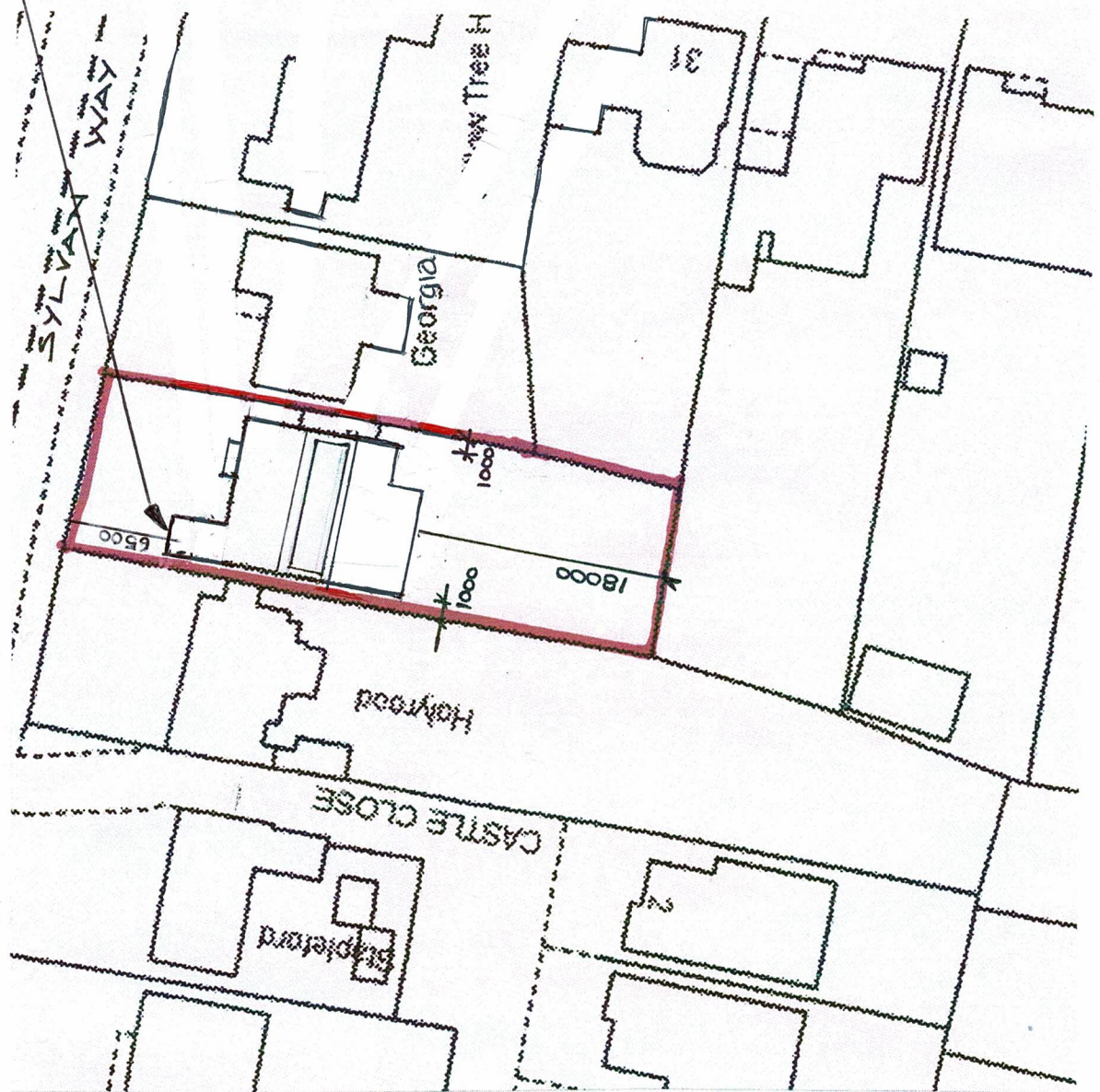
SITE PLAN 1:500
