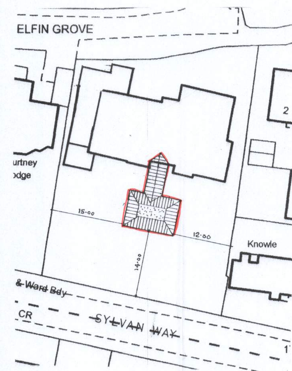
block plan 1 : 500
