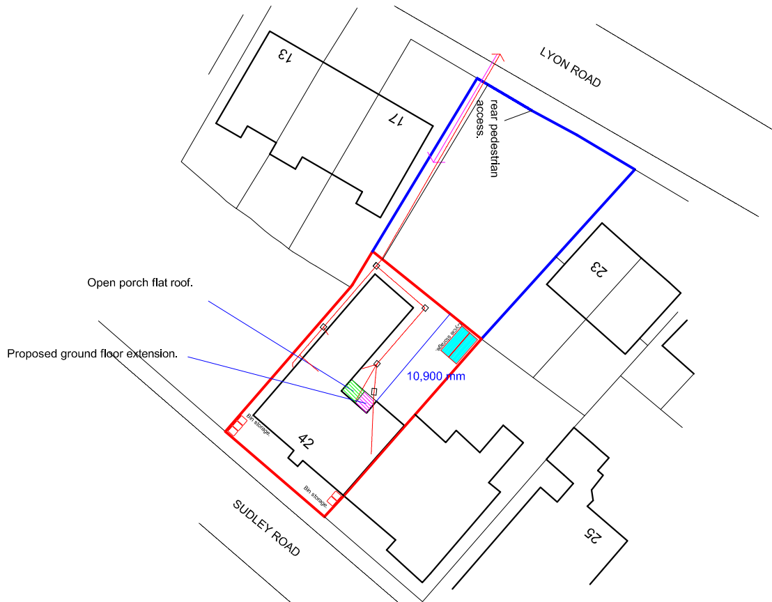
SITE PLAN - 1/500
