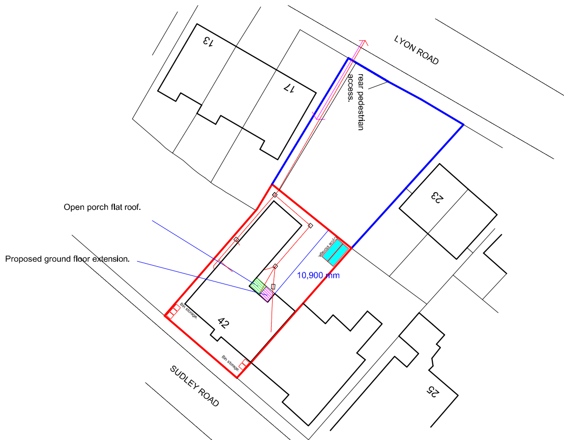
SITE PLAN - 1/500
