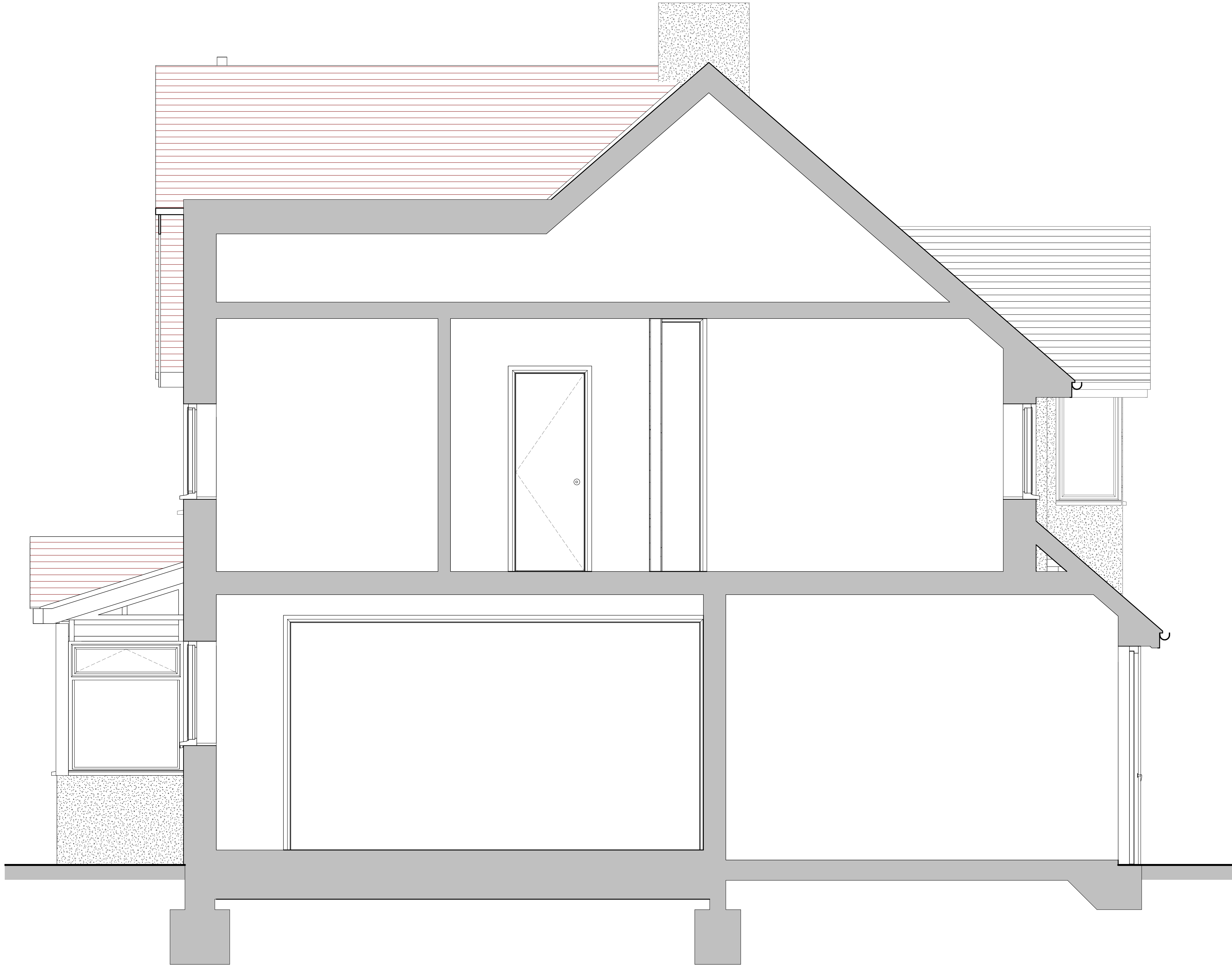
1 Section AA 1 : 20
