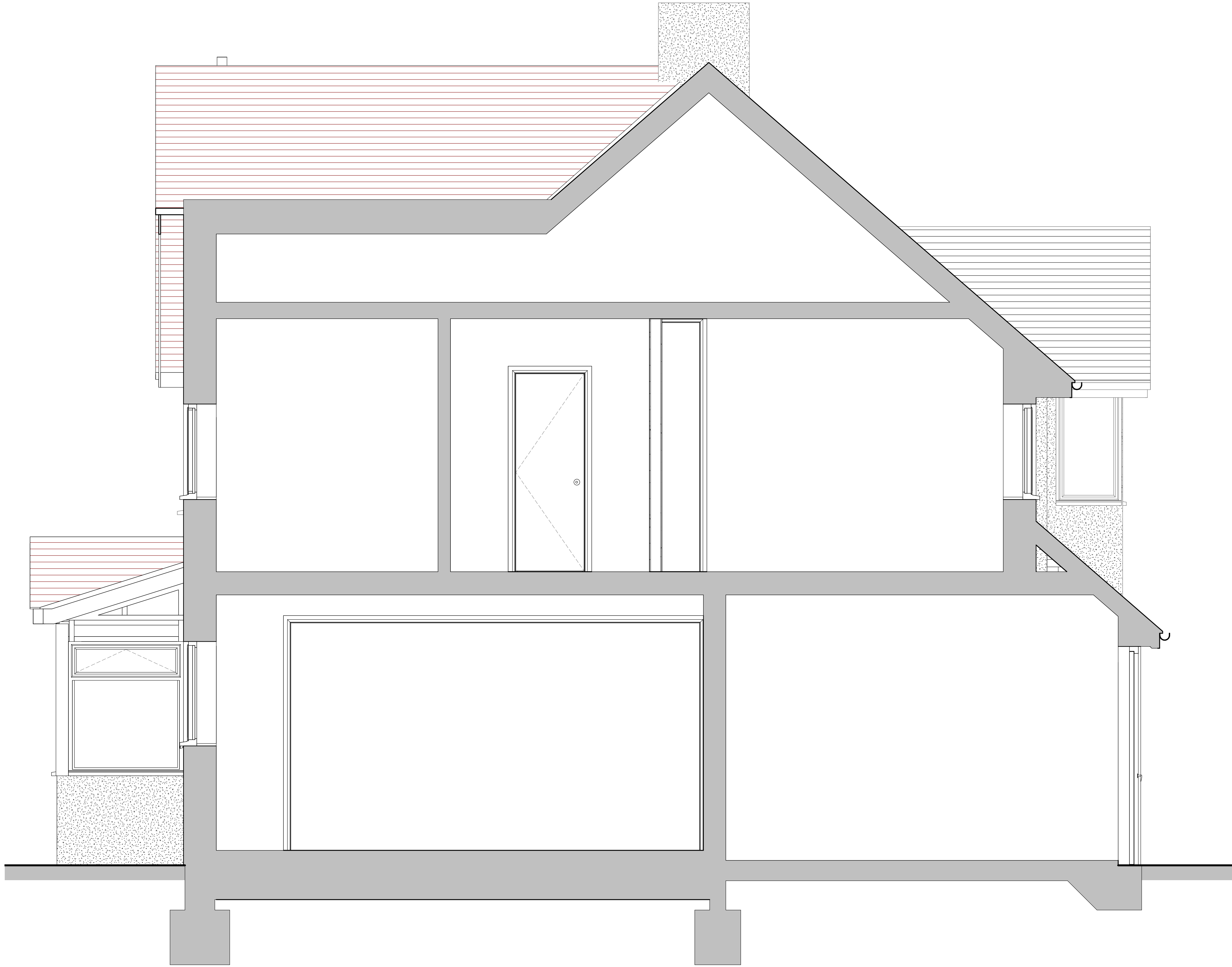
1 Section AA 1 : 20
