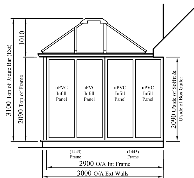
RIGHT ELEVATION
