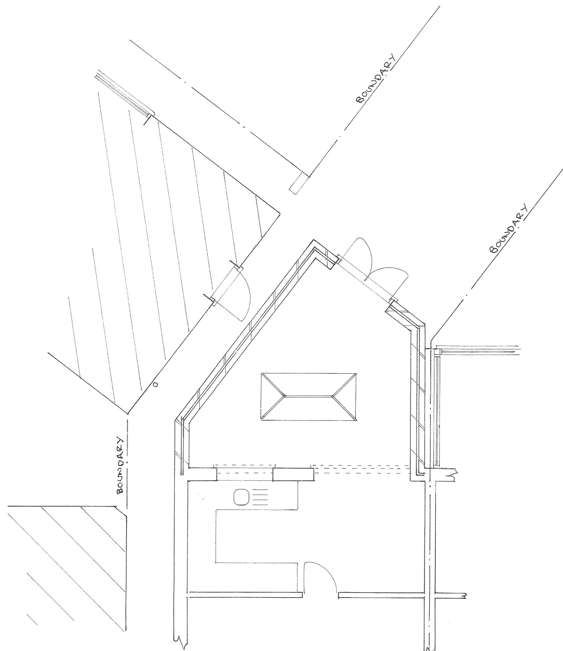
Plan 1 : 50
