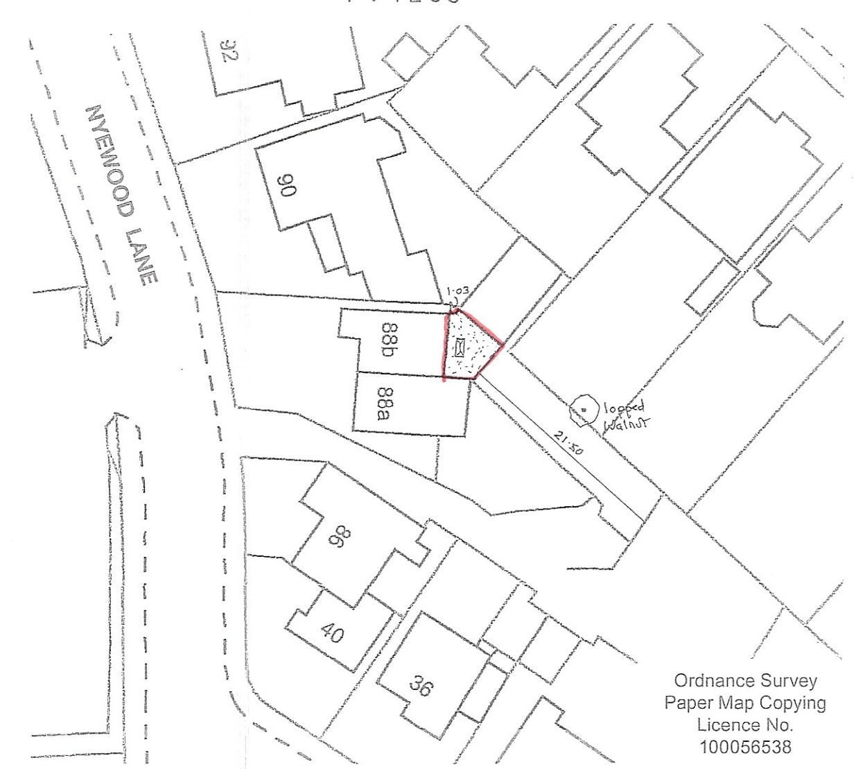
block plan 1 : 500
