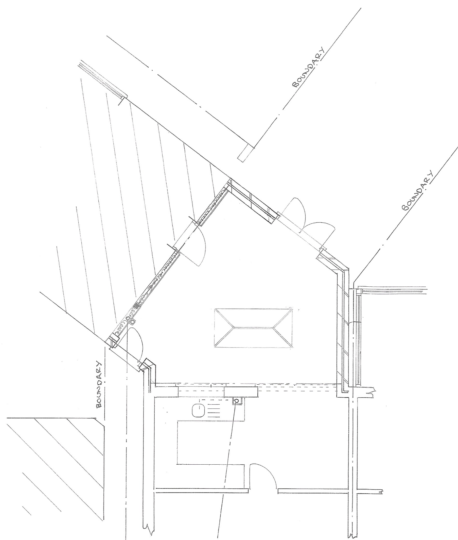
Plan 1 : 50
