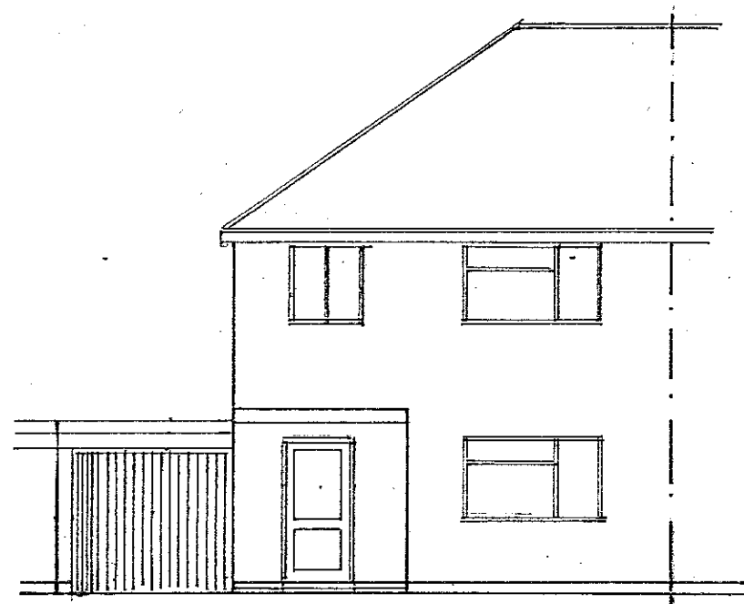
east 1 : 100
