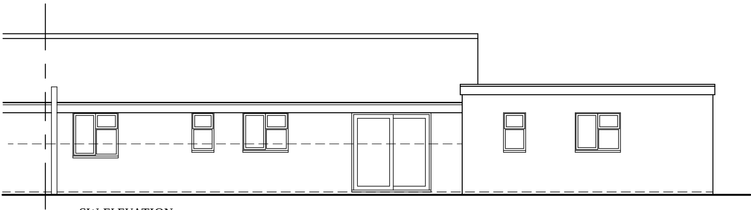
SW ELEVATION
