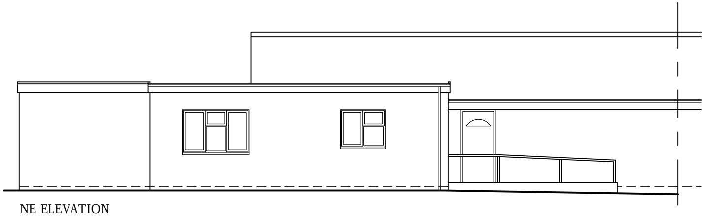
NE ELEVATION
