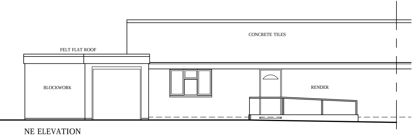
NE ELEVATION
