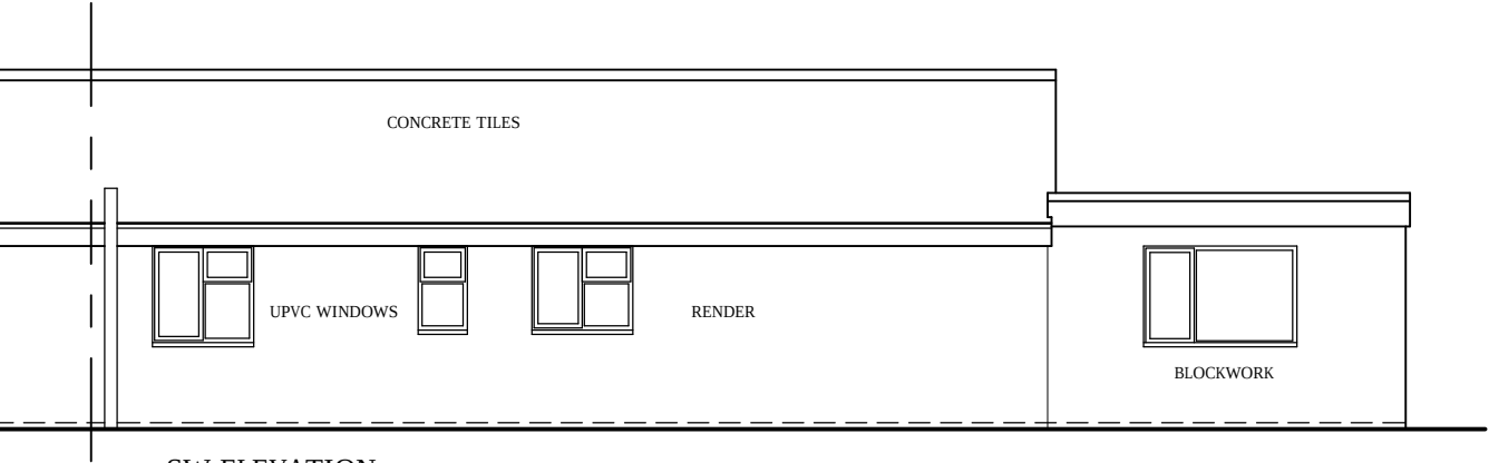
SW ELEVATION
