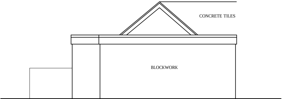
SE ELEVATION
