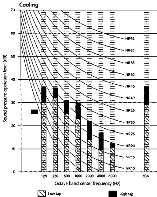
FCQG100F
