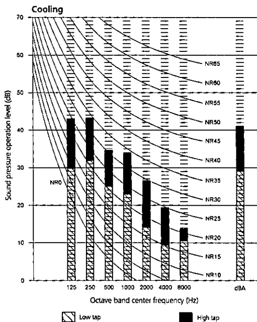
FCQG125-140F
