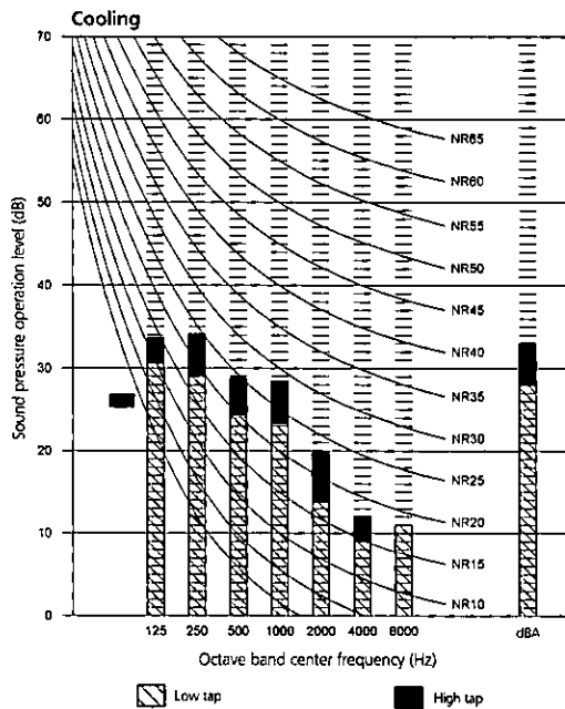
FCQG60-71F
