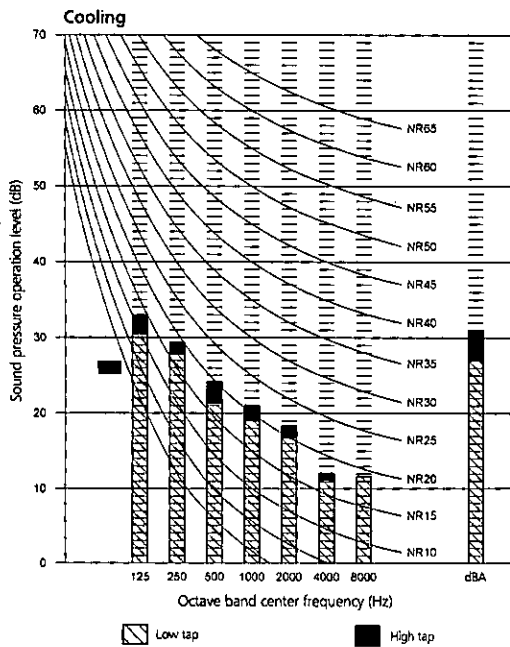
FCQG35-50F
