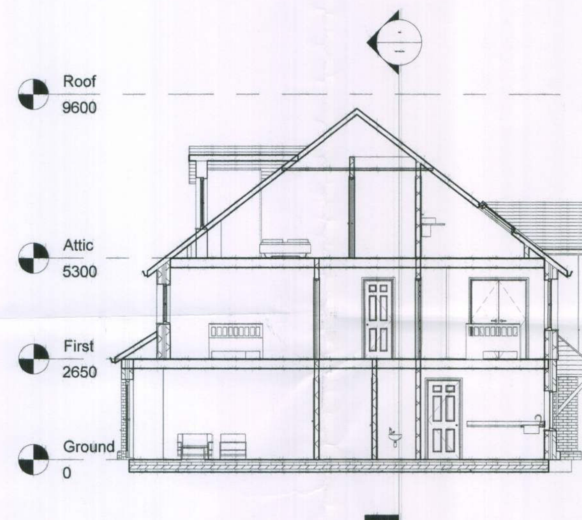
11 Section 1 1:100
