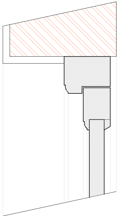
Door frame.
