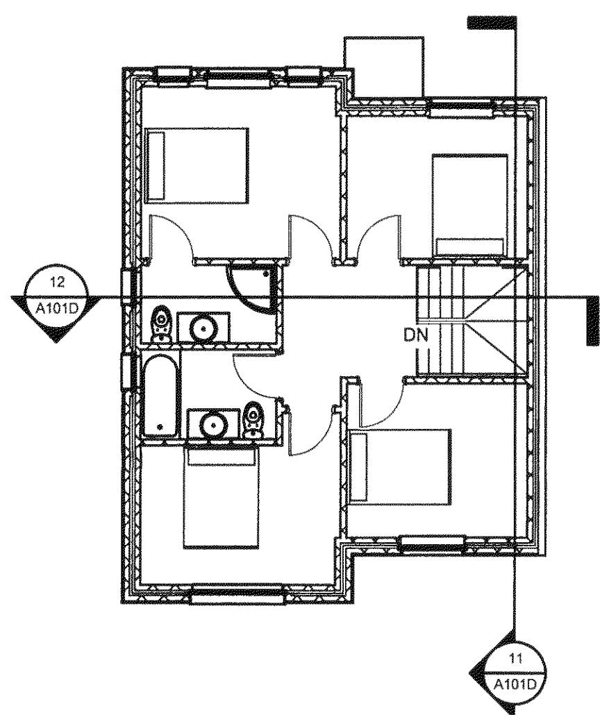
2 First 1 : 100
