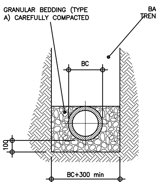
GRANULAR SIDE FILL
