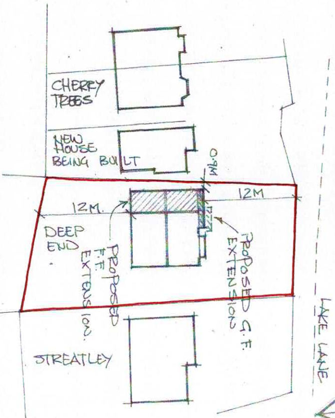
SITE PLAN 1:500
