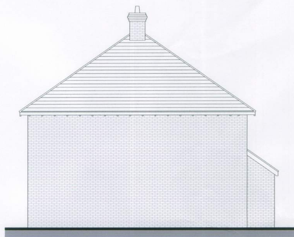
Elevation A
