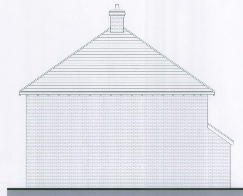
Elevation A
