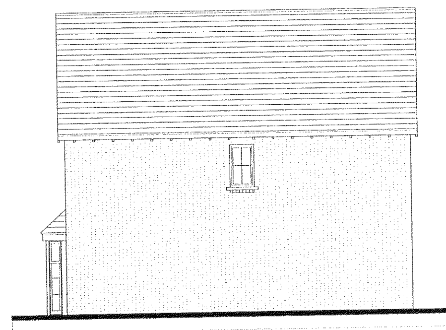
Elevation A
