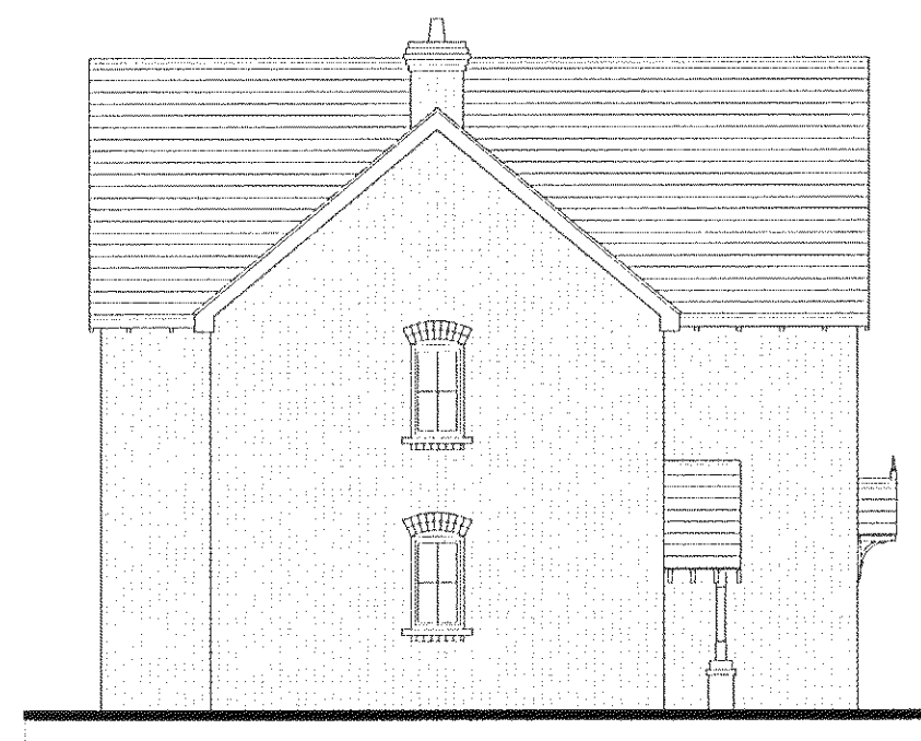
Elevation A
