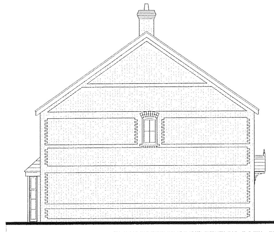
Elevation A
