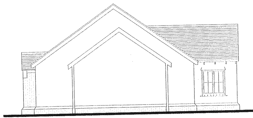
Elevation E
