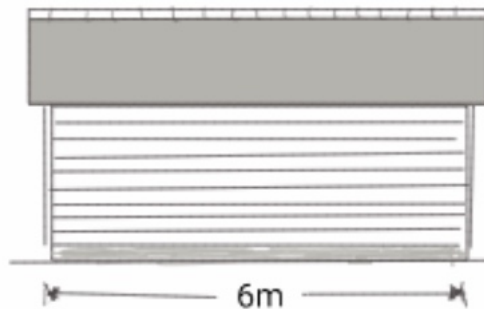
Right elevation
