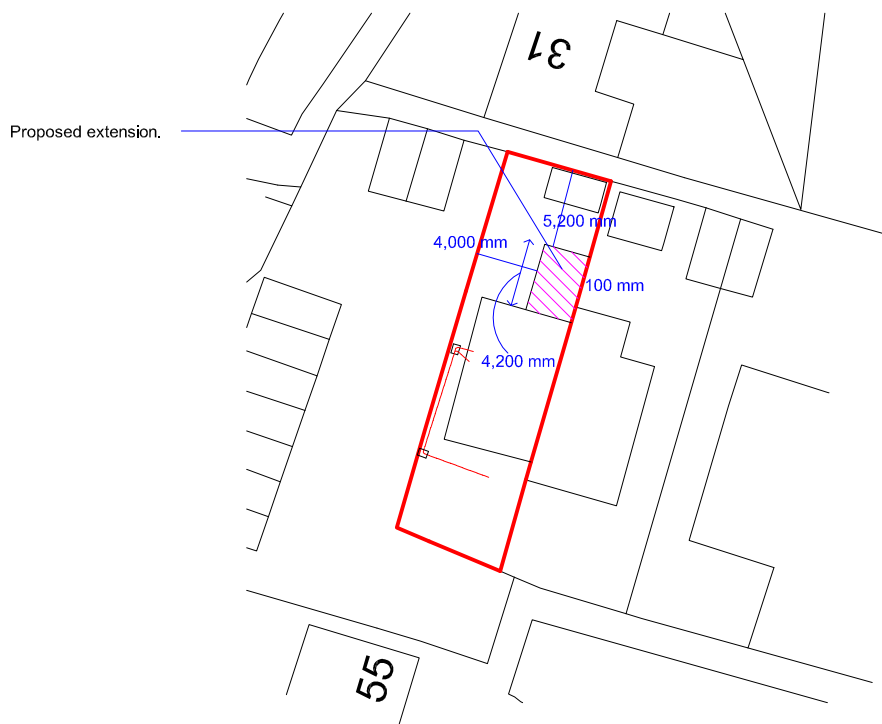
SITE PLAN - 1/500
