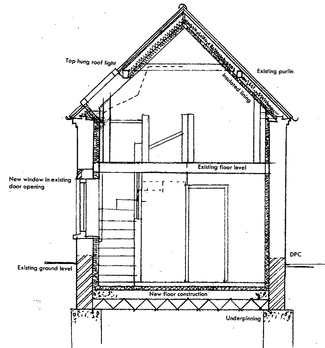
SECTION A-A
