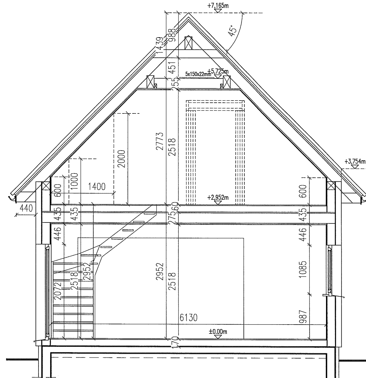
SECTION A-A
