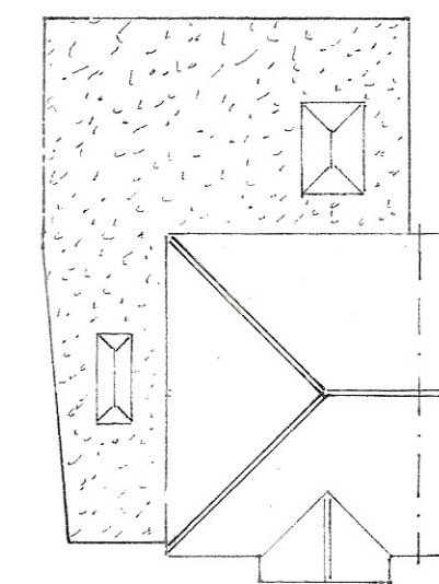
roof plan 1 : 200
