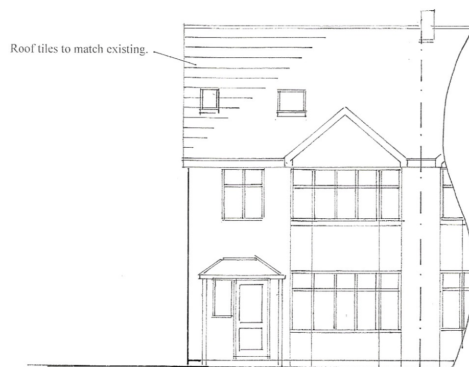
west 1 : 100
