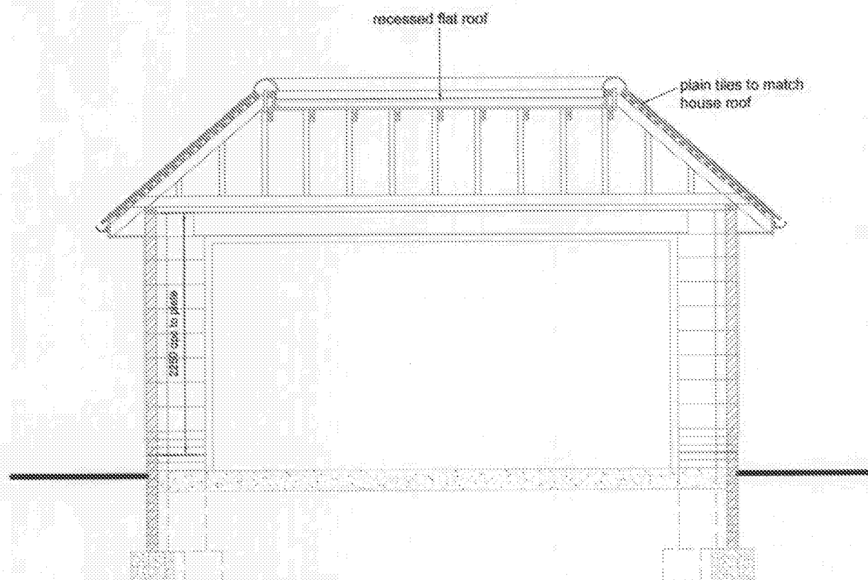
1:50 GARAGE SECTION A-A
