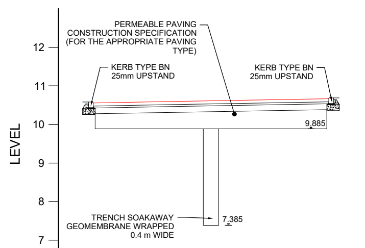
B-B SCALE: H 1:100,V 1:100. DATUM: 6.000
