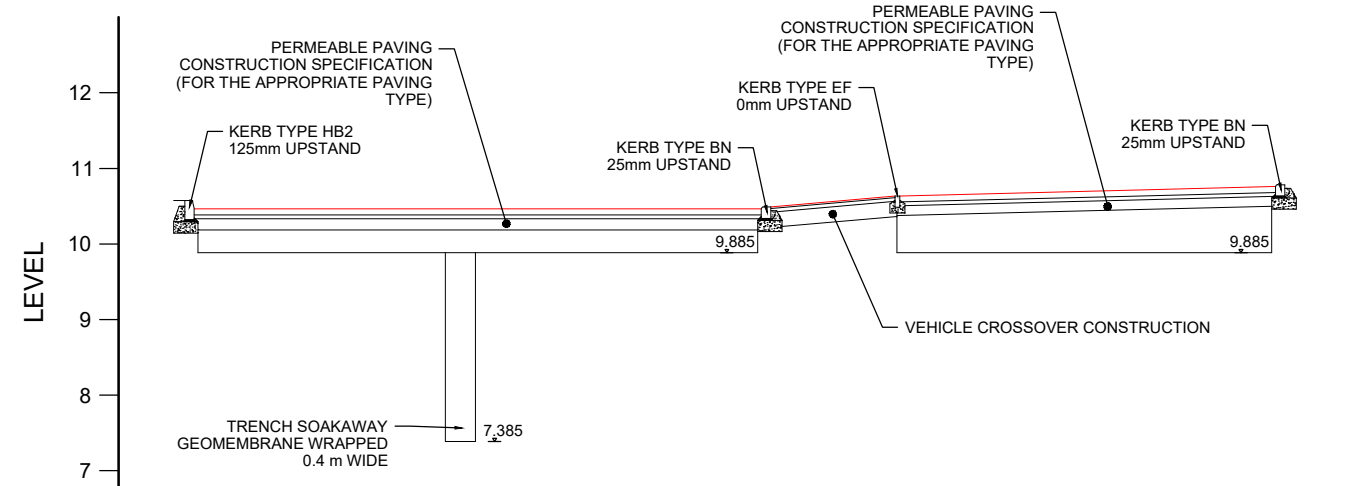
A-A SCALE: H 1:100,V 1:100. DATUM: 6.000
