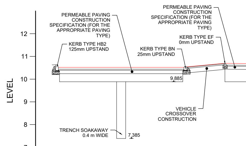
J-J SCALE: H 1:100,V 1:100. DATUM: 6.000
