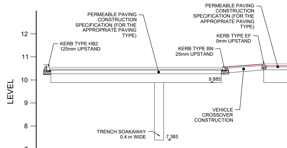
I-I SCALE: H 1:100,V 1:100. DATUM: 6.000
