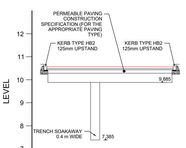
H-H SCALE: H 1:100,V 1:100. DATUM: 6.000
