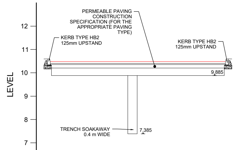
D-D SCALE: H 1:100,V 1:100. DATUM: 6.000
