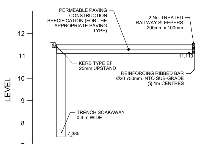
L-L SCALE: H 1:100,V 1:100. DATUM: 6.000
