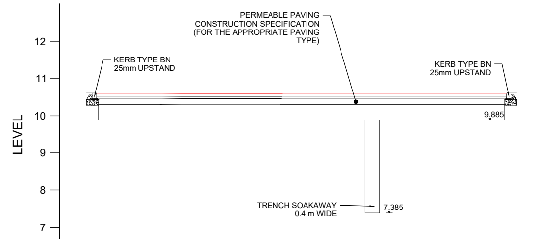
C-C SCALE: H 1:100,V 1:100. DATUM: 6.000
