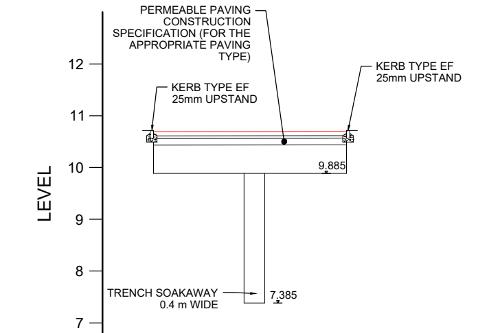
F-F SCALE: H 1:100,V 1:100. DATUM: 6.000
