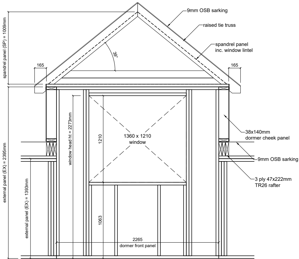
Dormer Elevation (Beds 3 & 4) (1:25)
