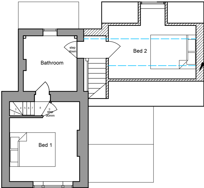
FF PLAN 1:100@A3
