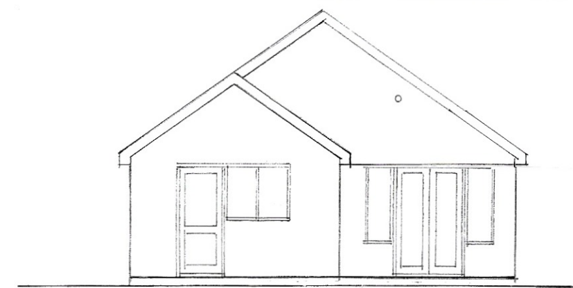
west 1 : 100
