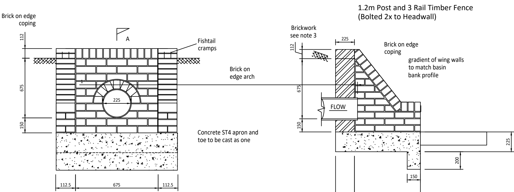
Elevation
