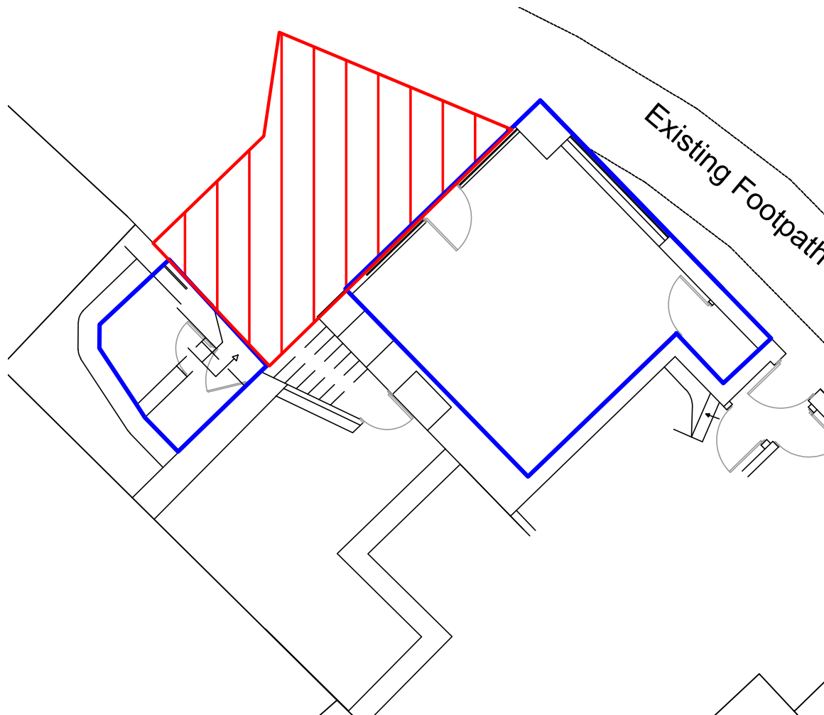
Site Plan 1:100
