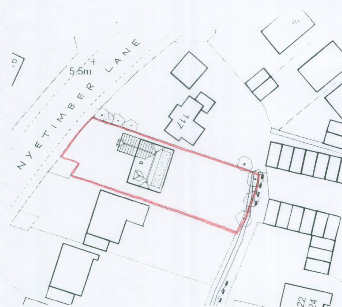
block plan 1 : 500
