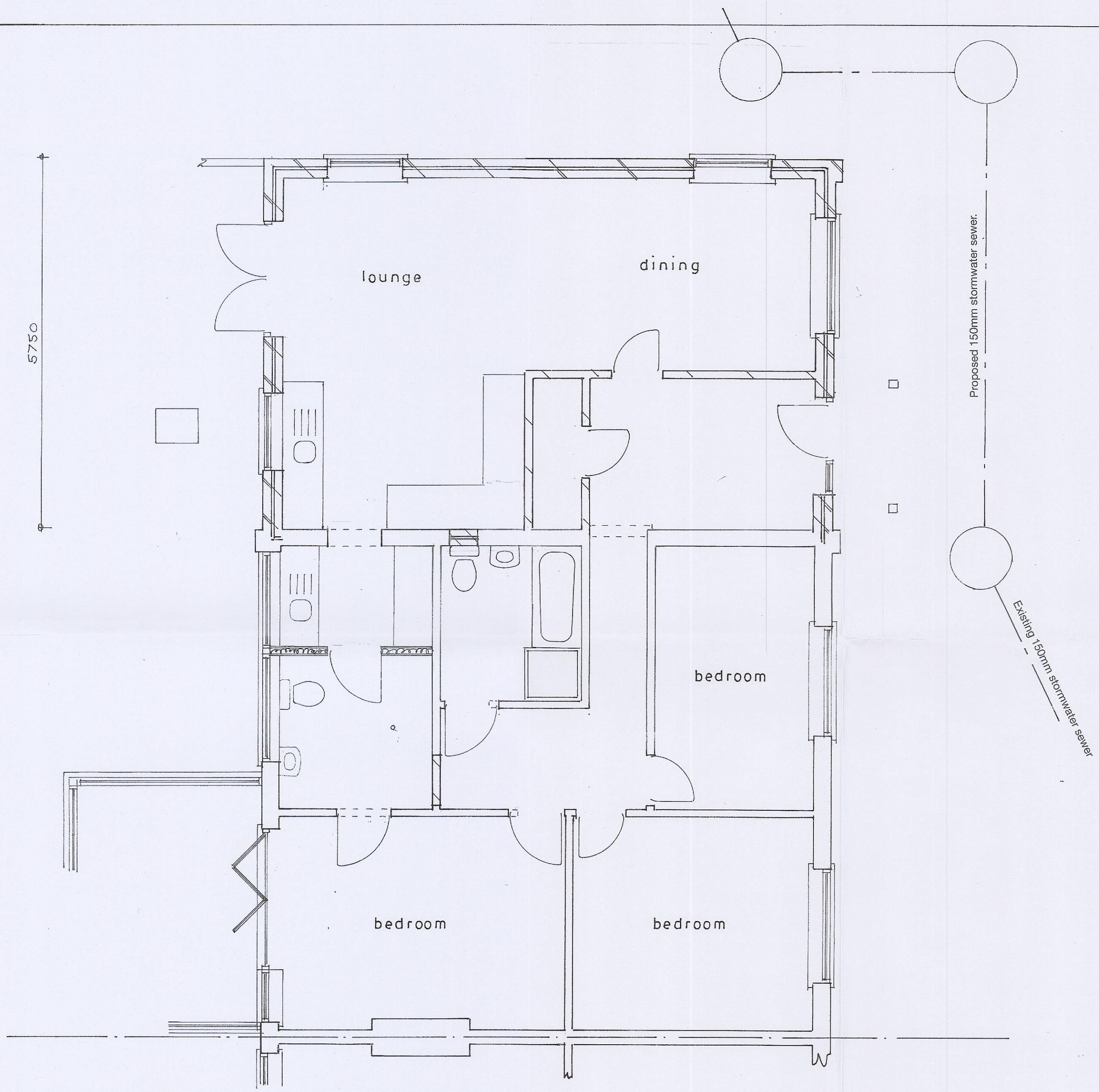
Plan 1 : 50
