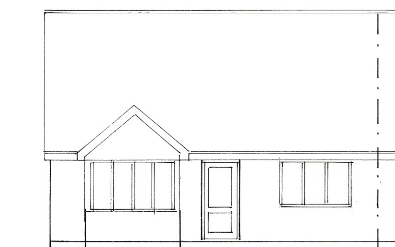
east 1 : 100
