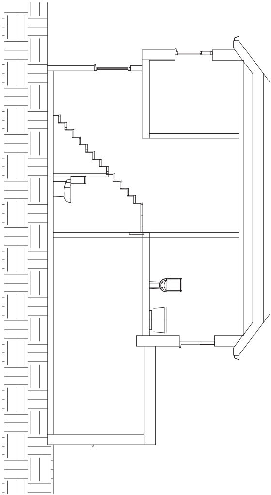
Section A-A
