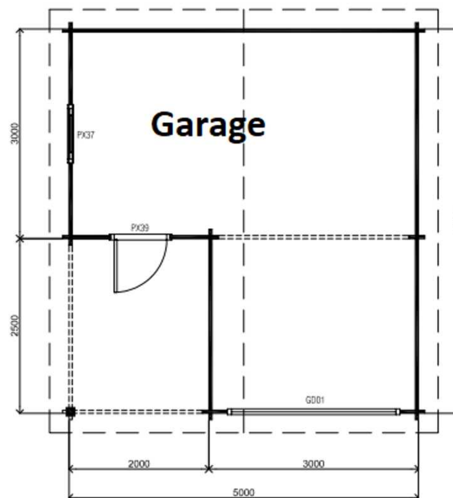
Plattegrond / Plan
