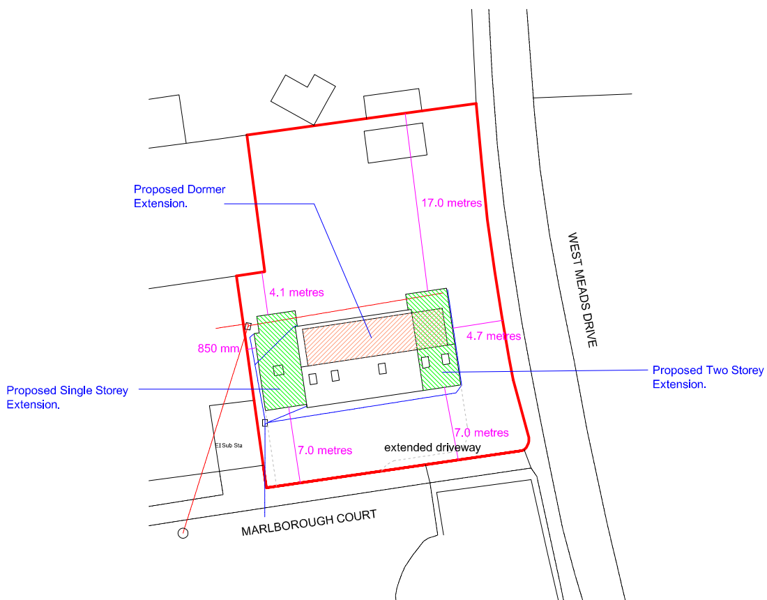
SITE PLAN - 1/500
