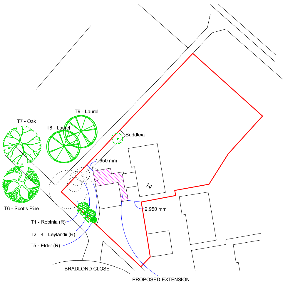
SITE PLAN - 1/500
