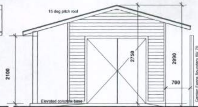
Elevation B-B 1:50
