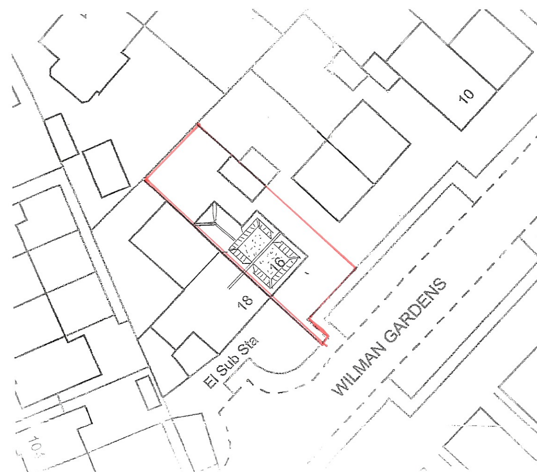
block plan 1 : 500
