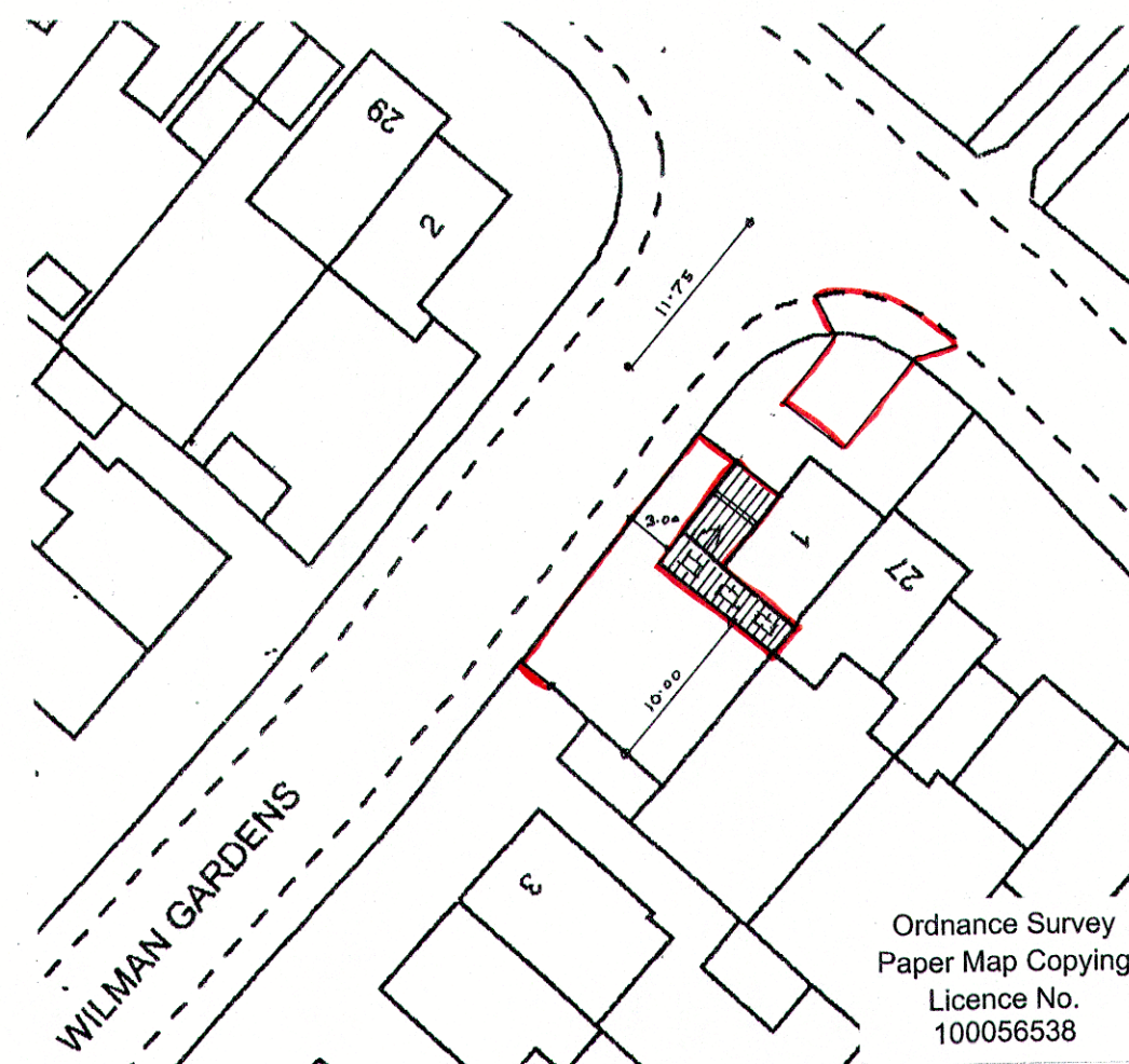
block plan 1 : 500
